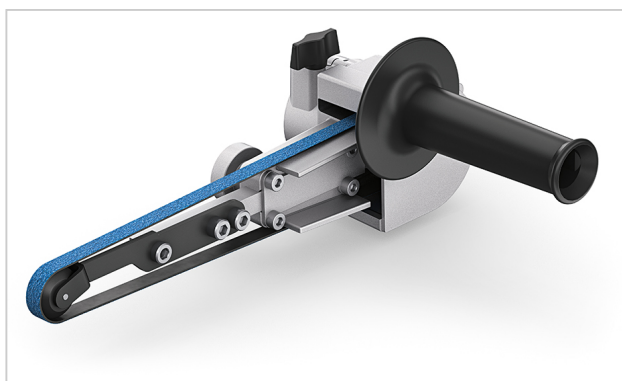
Nástavec pásového pilníku na TRINOXFLEX. Upevnitelný bez nástrojů rychlo-výměnným systémem. Včetně brusných ramen 9 a 30 mm, postranní
